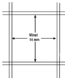
Alternativ 2 Fyrkantmaskor
