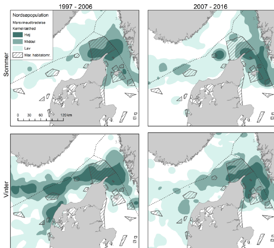
Figur 10 Tæthet (kärnområdesdensitet) av tumlare försedda med satellitsändare inom Nordsjøpopulationens förvaltningsområde fördelat på två tio-årsperioder samt säsong. Kärnområdeskategorierna är hög (minsta möjliga område som rymmer 30 % av alla tumlarpositioner, medel (31–60 %) respektive låg (61–90 %). Antal tumlare och positioner per analys år: 1997–2006 april–september: 18 djur/906 positioner; 1997–2006 oktober–mars: 32 djur/817 positioner; 2007–2016 april–september: 27 djur/799 positioner; 2007–2016 oktober–mars: 28 djur/1004 positioner. Figur från Sveegaard et al. (2018).
