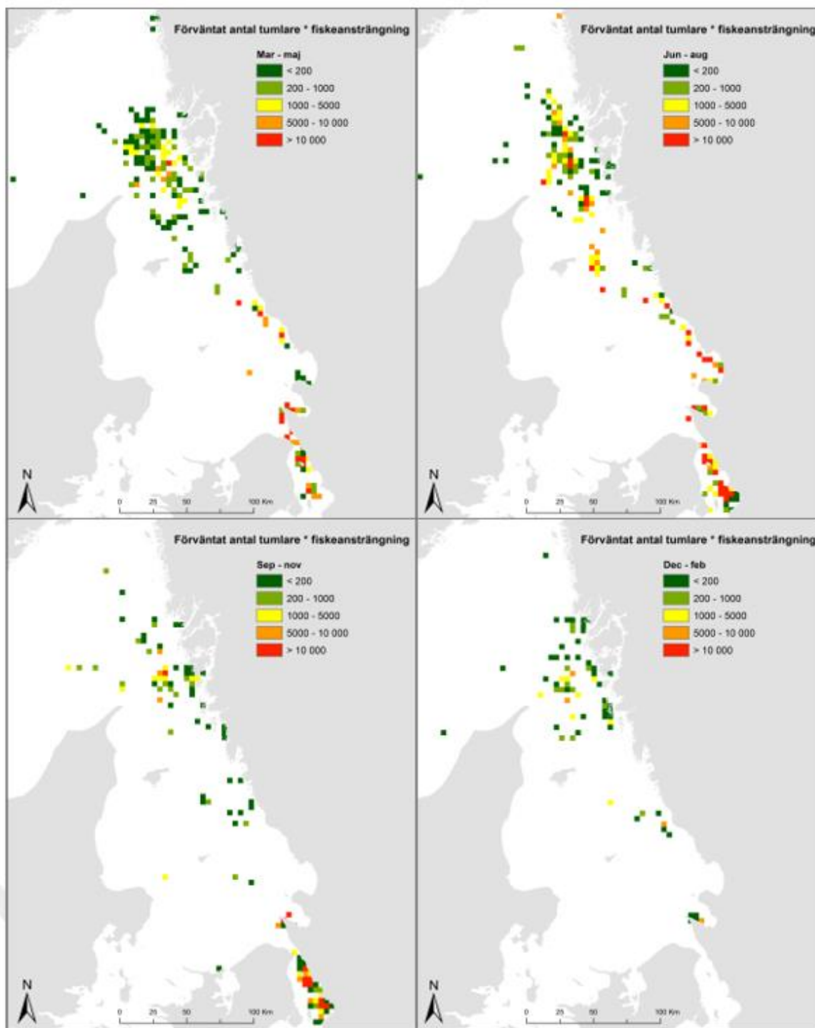
Figur 13 Bifångstrisk för tumlare i Västerhavet beräknad genom att multiplicera data om tumlartäthet från satellitmärkta tumlare under perioden 1997–2008 (data från Aarhus universitet, Danmark) med rapporterad fiskeansträngning med passiva nätredskap (sillnät exkluderade) under 2015 (Havs- och vattenmyndigheten). Bifångstrisken anges som ett relativt index och visar i vilka områden risken för bifångst är högre alternativt lägre relativt till varandra. Skalan i kartorna över Västerhavet kan inte jämföras med skalan i kartorna över Östersjön.
