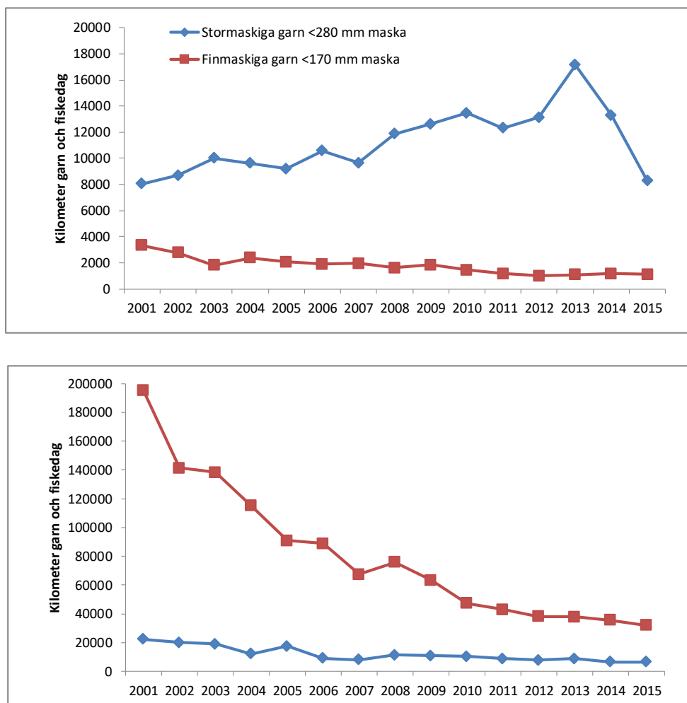
Figur 8 Summa av fiskeansträngning från svenskt fiske. Blå linje representerar fiske med grimgarn, skäddegarn, tungegarn, laxdrivgarn, piggsvars garn och laxgarn. De maximala maskstorlekarna för detta fiske ligger mellan 180 to 280 mm (diagonalmaska). Röd linje representerar fiske med öring, krabba, torsk, bleke, hajgarn samt gös, aborre, sik och gäddnät. De maximala maskstorlekarna ligger mellan 80 och 170 mm (diagonalmaska) i (A) Skagerrak och Kattegatt respektive (B) Östersjön söder om 60°N från 2001 till 2015.
