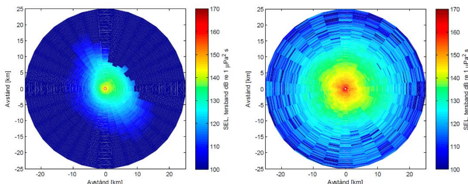
Figur 9 Beräknad ljudexponeringsnivå (2 kHz, 1/3 oktavband) runt en pålning (källstyrka 197 dB re 1 µPa²s) i augusti i Kattegatt (vänster) respektive södra Östersjön (höger). Det mörkblå området i bäringsintervallet från -20° till 135° i Kattegatt utgörs av land. Figur från (Andersson et al., 2016).
