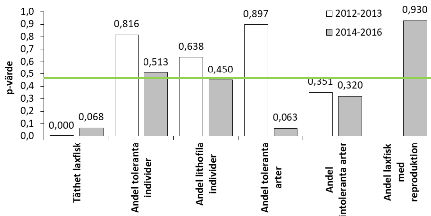
Figur 3. Redovisning av de sex ingående parametrarna i VIX för bedömning av generell påverkan på elfiskeloken "Tingebro" i Emån under perioden 2012-2013 respektive 2014-2016. Den heldragna gröna linjen markerar den nedre gränsen för god status (0,467). Dataetiketterna avser medelvärdet för respektive parameter och period.
