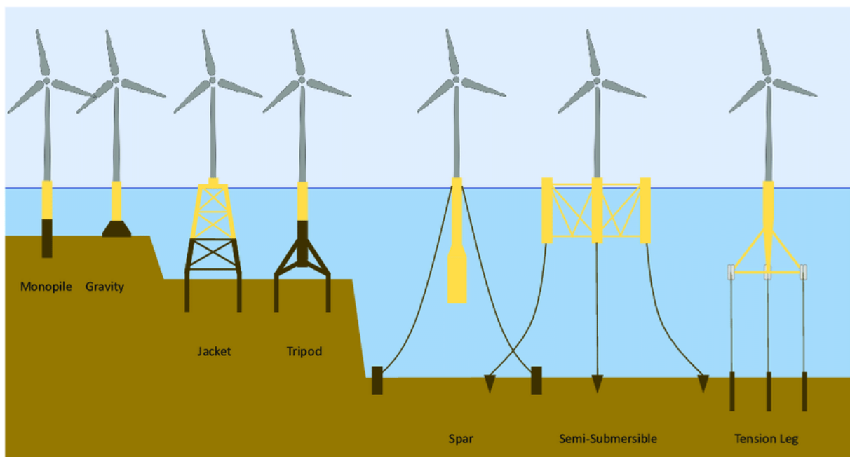
Figur 6-5 Olika fundamentstyper, från vänster: Monopile, gravitation, fackverk, trefot, boj, halvnedsänkt och TLP (Dornhelm, Seyr, och Muskulus 2019) cc-by
