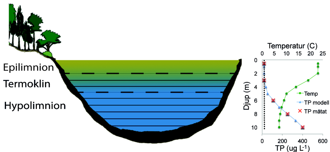
378 379 Figur 1: 380 Skiktad, dimiktisk sjö (vänster) och profildata för temperatur och totalfosfor (TP) (höger). 381 Horisontella streckade linjer i sjön representerar gränser för termoklinen. Den vertikala streckade 382 linjen representerar bakgrundhalten av TP (20 ug/L i detta exempel) som subtraheras från alla TP- 383 koncentrationer i profilen innan P-massan beräknas.
