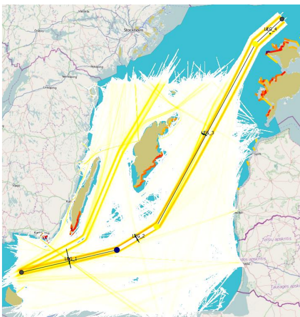
Figur 11. Resultat av IWRAP-beräkning av kollision- och grundstötningssannolikhet för omdirigeringsalternativ 1, djupvattenleden.
