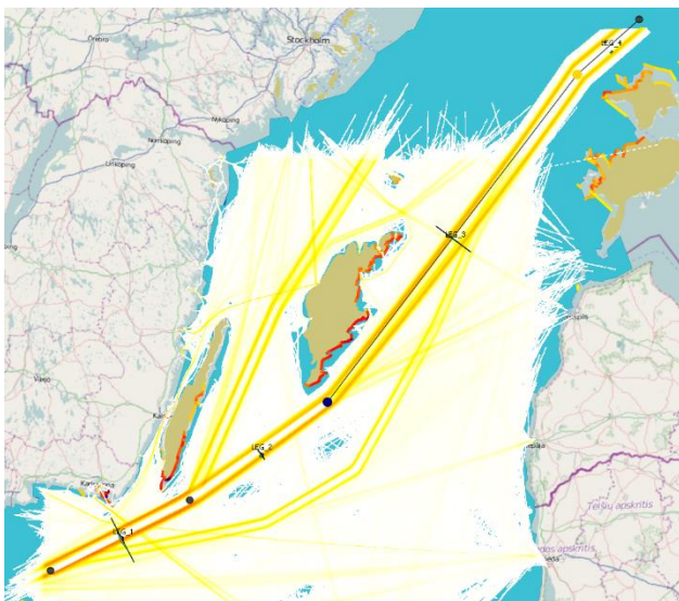
Figur 10. Resultat av IWRAP-beräkning av kollision- och grundstötningssannolikhet för nulägesbildens trafiksituation.
