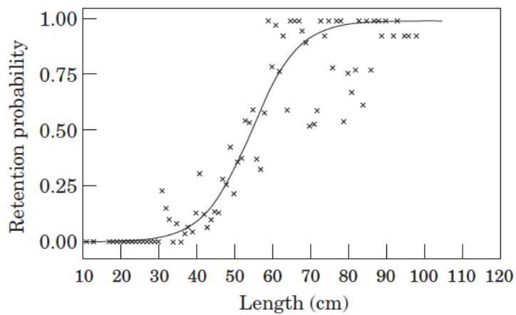
Figur 2. Selektivitet i bottentrål med 140 mm maska för torsk (från Huse m.fl. 2000).
