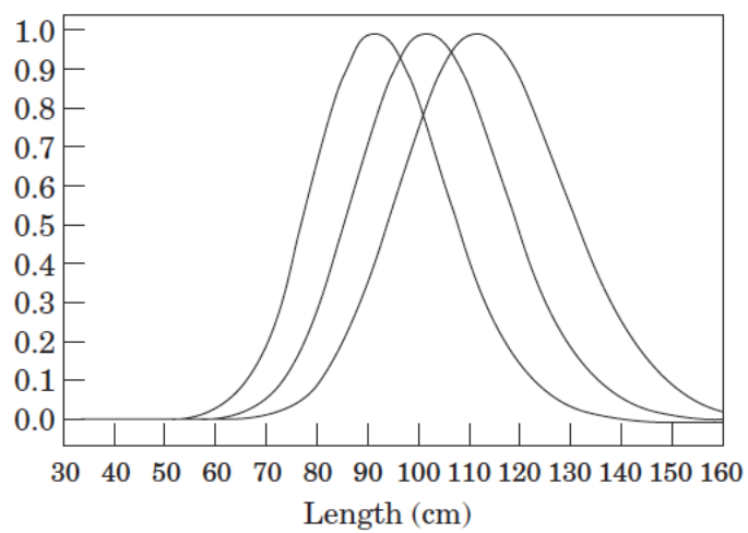
Figur 3. Selektivitet i torskgarn med 186, 200 eller 220 mm maskstorlek för torsk (från Huse m.fl. 2000).
