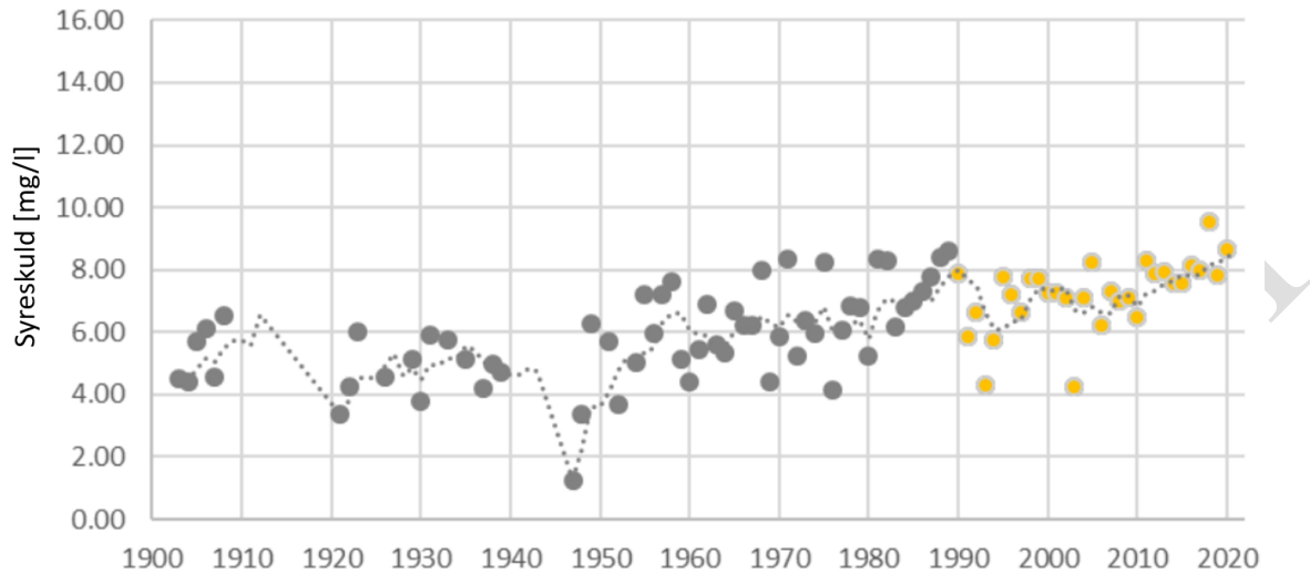
Figur 1 Syreskuldutveckling med tid i Bornholmshavet och Hanöbukten. Punkterna sedan 1990 visar en signifikant försämring (Mann-Kendall test, p < 0,05 ). Från HELCOM 2023c
