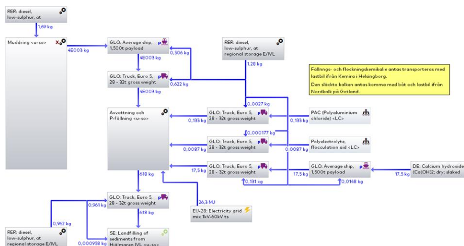
Figur 17 Processflöde för LCA konventionell muddring
