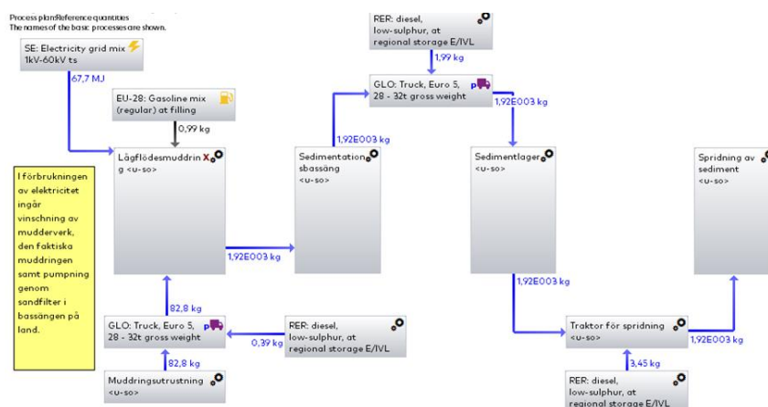
Figur 18 Processflöde för LCA lågflödesmuddring.
