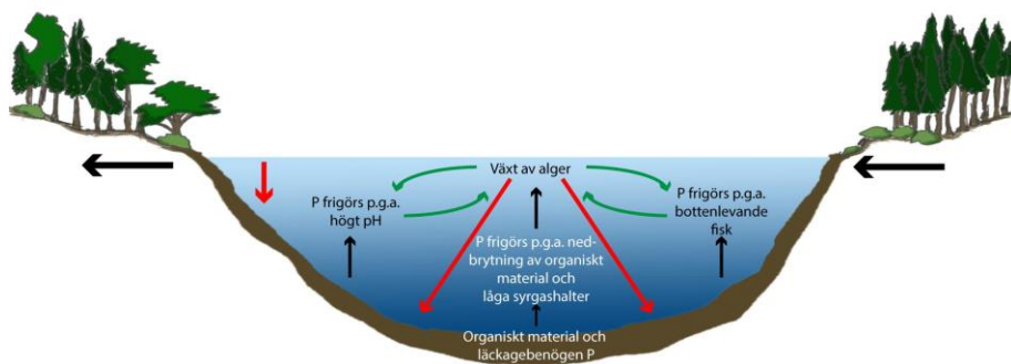
Figur 13 En förenklad version av fosforkretsloppet i helt omblandade och polymiktiska, svagt skiktade kustvikar. De svarta linjerna visar bruttointernbelastning, de röda sedimentation av fosfor och de gröna algernas användning av fosfor från interna källor (bildkälla Huser 2021) 46 .
