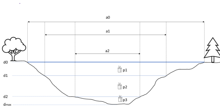
Figur 12. Schematiskt tvärsnitt av sjö som visar den totala arean ( a_0...a_2 ) vid olika djup ( d_0...d_{max} ). p_1...p_3 anger provtagningsplatser inom djupintervallen.
