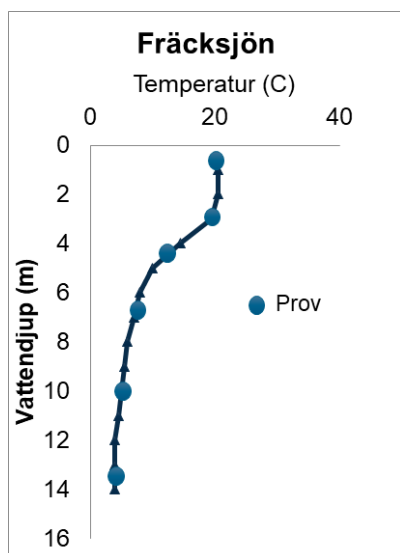
Figur 7. Temperaturprofil vid skiktning i Fräcksjön samt djup för provtagningar.
