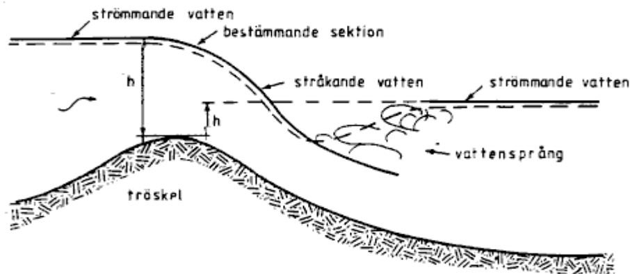
Figur 1. Bestämmande sektion. ( h nedströms < 2/3 * h uppströms)
