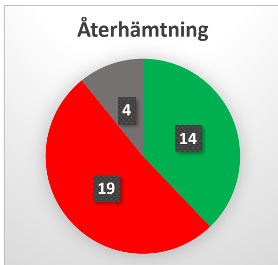
Figur 2. Summering av utveckling för känsliga fiskarter på Nordsjökala i relation till de två bedömningskriterierna: (vänster) arter som når tröskelvärde för återhämtning. Resultaten baserar sig på en integrerad bedömning av flera olika provfisker i Nordsjön enligt Oskar.
