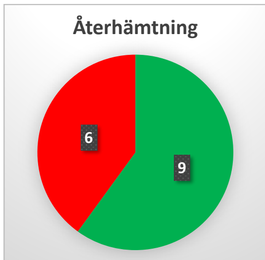
Figur 1. Summering av utveckling för känsliga fiskarter på Västerhavsskala i relation till det primära bedömningskriteriet: antal arter som når tröskelvärdet för återhämtning. Bedömning baserar sig på provfisket IBTS kvartal 1 i Västerhavet 1983–2020.
