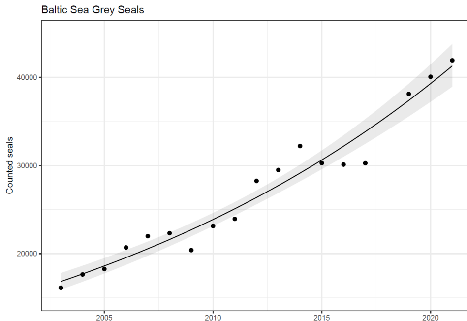
Figur 1. Antalet räknade sälar i Östersjön vid de årliga inventeringarna under pälsbytet åren 2003–2021. Andelen sälar på land uppskattas till 70 % av den totala populationen. Den årliga tillväxten under perioden 2003–2021 var 5,1 % med 80 % stöd för en tillväxt på \geq 4,7 % vilket är under tröskelvärdet på 7 %. Tillväxthastigheten visar inga tydliga tecken på att avta vilket tyder på att populationen inte påverkas av täthetsberoende faktorer och därmed fortsatt är under TRL. Modellerat index för antal räknade sälar (svart linje) med 95% konfidensintervall (grå skuggning).
