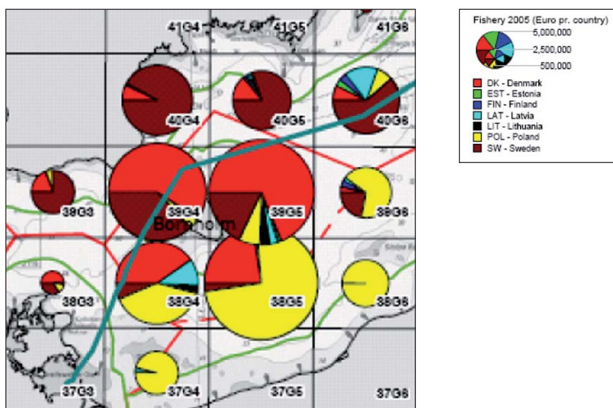
Fig. 11. Fångstvärde per land i Hanöbukten 2005. Källa: Underlagsmaterial från Nordstream. Den gröna linjen som går snett uppför från höger ner till fastlandet i Tyskland i kartorna är den tänkta sträckningen för gasledningen mellan Ryssland och Tyskland.
