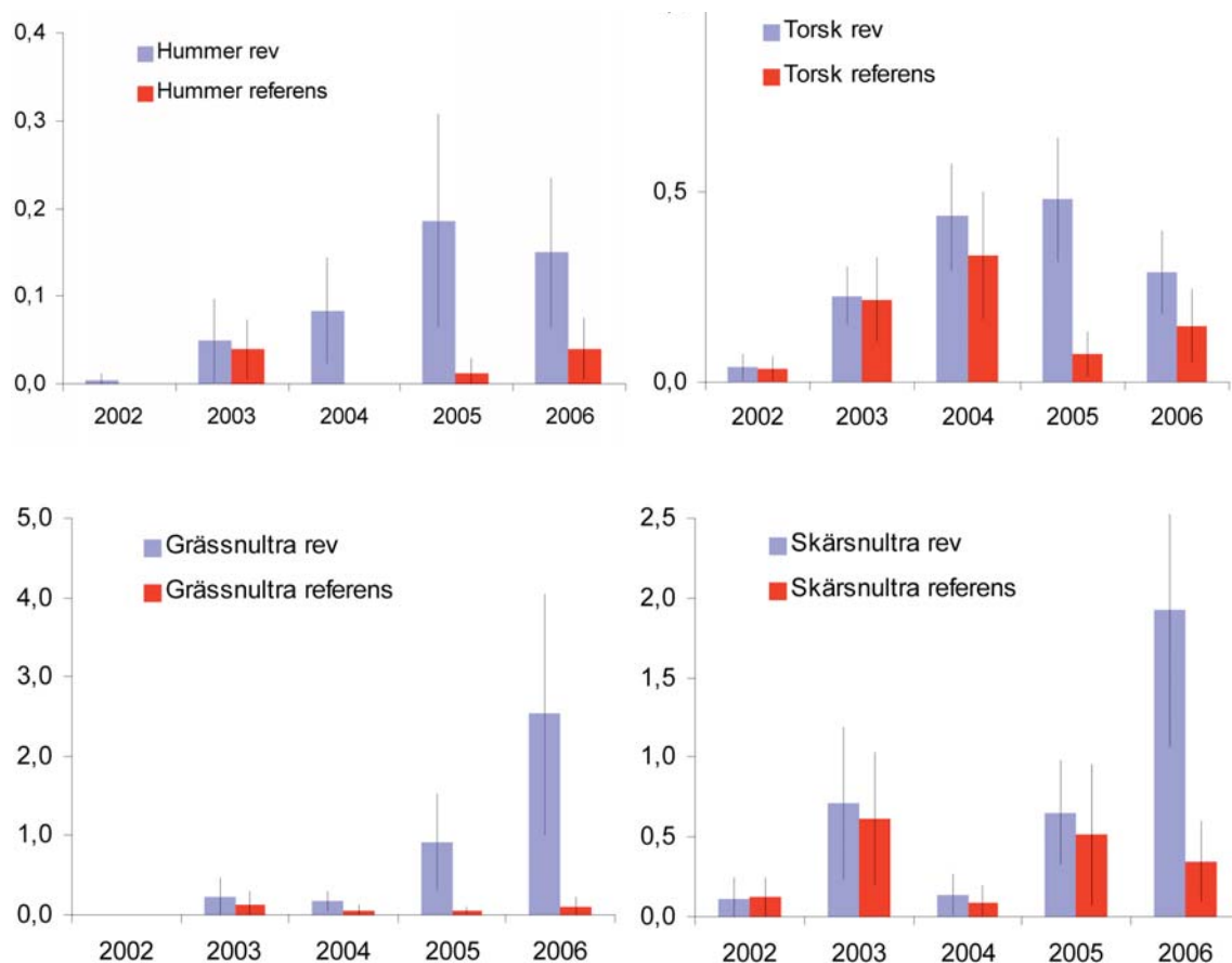
Fig. 19. Fångst per ansträngning (per ryssjehus och dygn) av hummer, torsk, grässnulta och skärsnulta i ryssjefiske vid konstgjorda reven och i referensområden 2002–2006.
